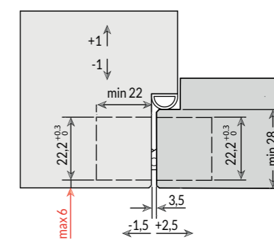
Sezione porta raso con battuta Rebated flush door cross-section Sección puerta enrasada y solapada
