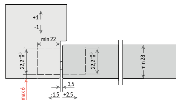
Sezione porta raso senza battuta Unrebated flush door cross-section Sección puerta enrasada
