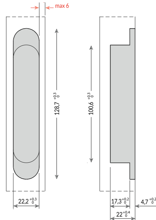
Misure della cava Slot measurement Medidas de corte
